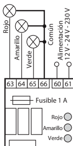
(Opcional: tarjeta semáforo de empalme para lámparas de 230 V) cód. 7282L
